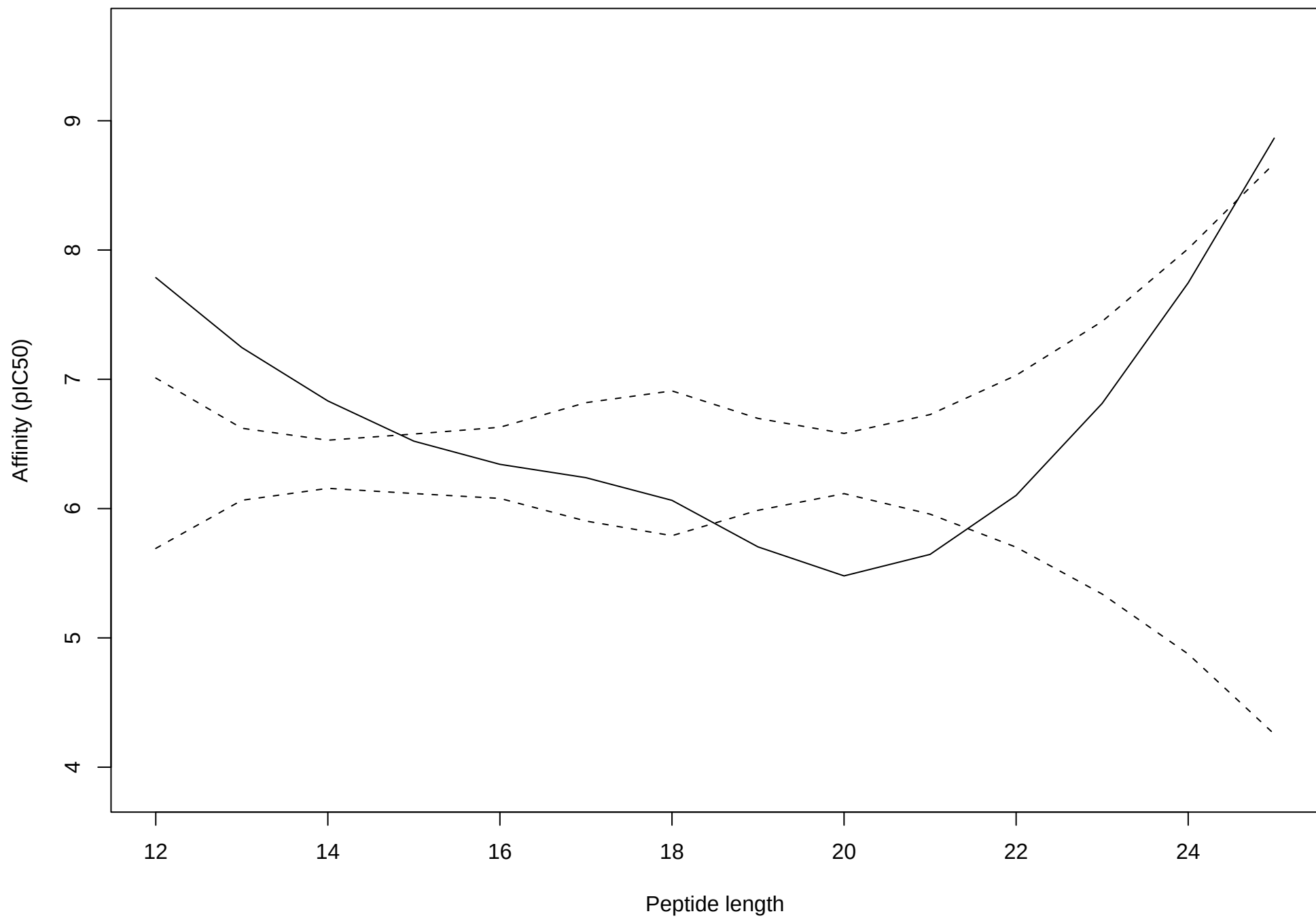
DRB1*0101 local regression fit
